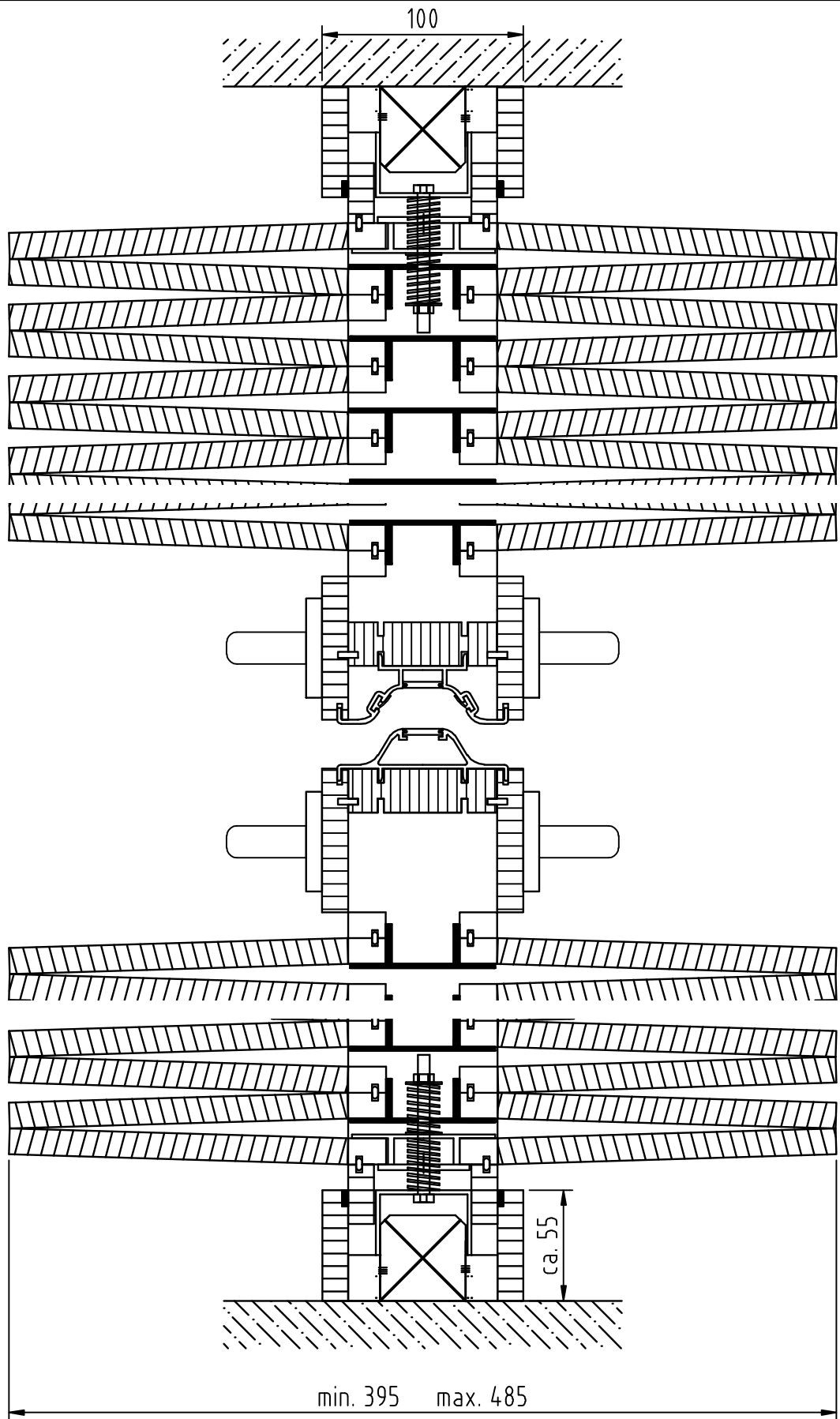
Paketbreite in Abhängigkeit von Öffnungsbreite und Anzahl der Lamellenpaare
