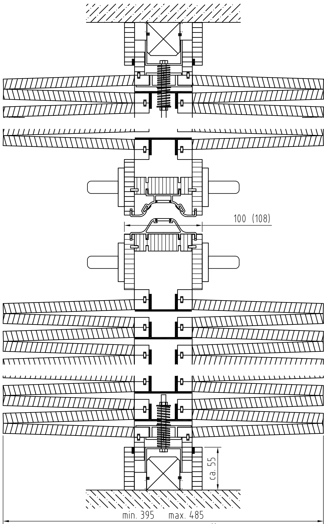
Paketbreite in Abhängigkeit von Öffnungsweite und Anzahl der Lamellenpaare
